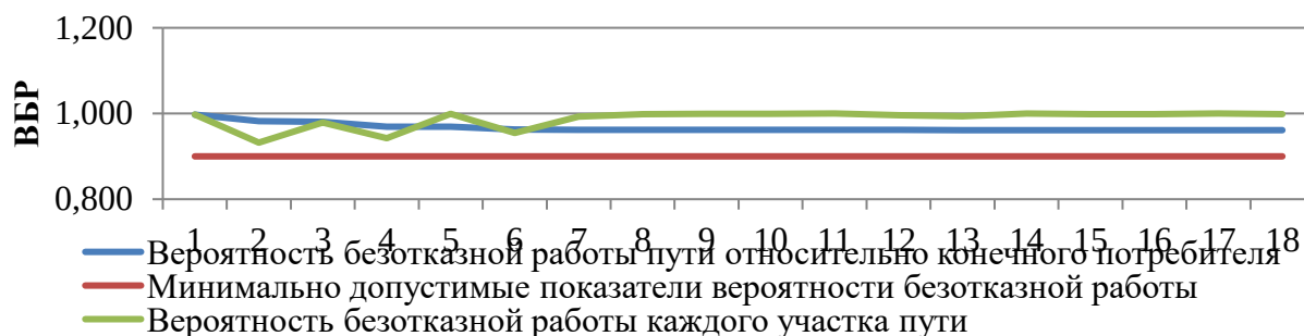
Рисунок 69. ВБР относительно участка тепловой сети от камеры «Вывод - Котельная № 9» до потребителя по ул. Заводская, 11
