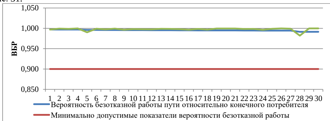
Рисунок 31. ВБР относительно участка тепловой сети от камеры «Вывод - Котельная № 5» до потребителя по ул. Семакова, 58
