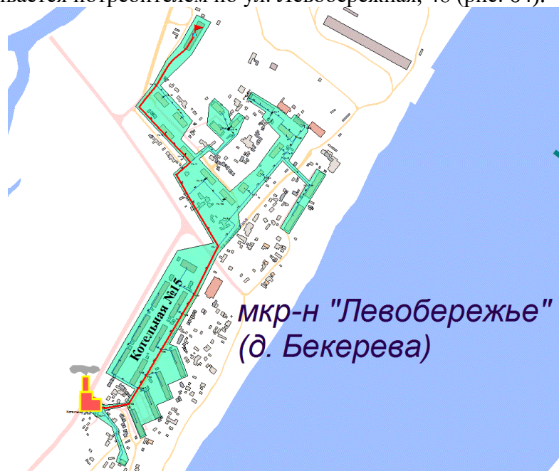
Рисунок 64. Трассировка участка тепловой сети от камеры «Вывод - Котельная № 15» до потребителя по ул. Левобережная, 48
