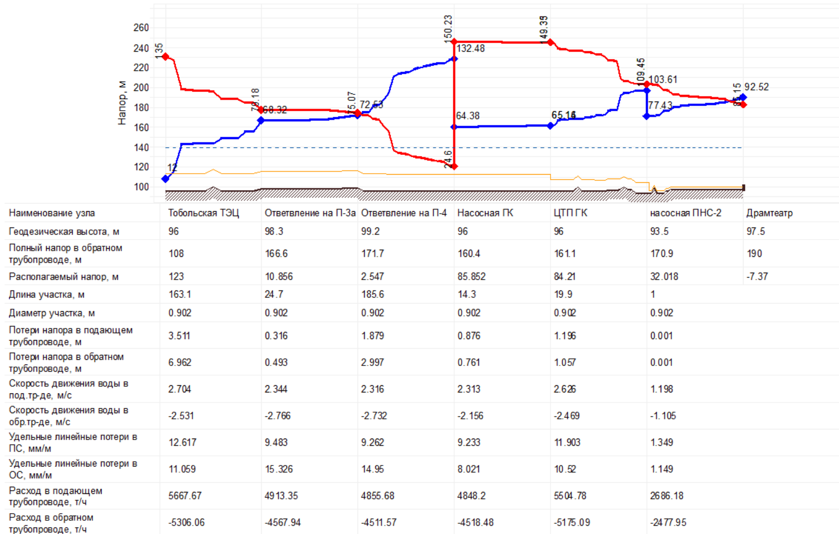
Рисунок 22. Пьезометрический график тепловой сети от ЭТПГ до потребителя «Драмтеатр»
