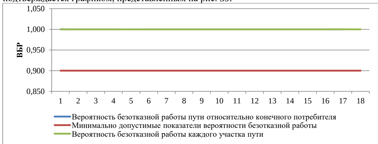
Рисунок 39. ВБР относительно участка тепловой сети от камеры «Вывод - Котельная № 12» до потребителя по ул. Гоголя, 41
