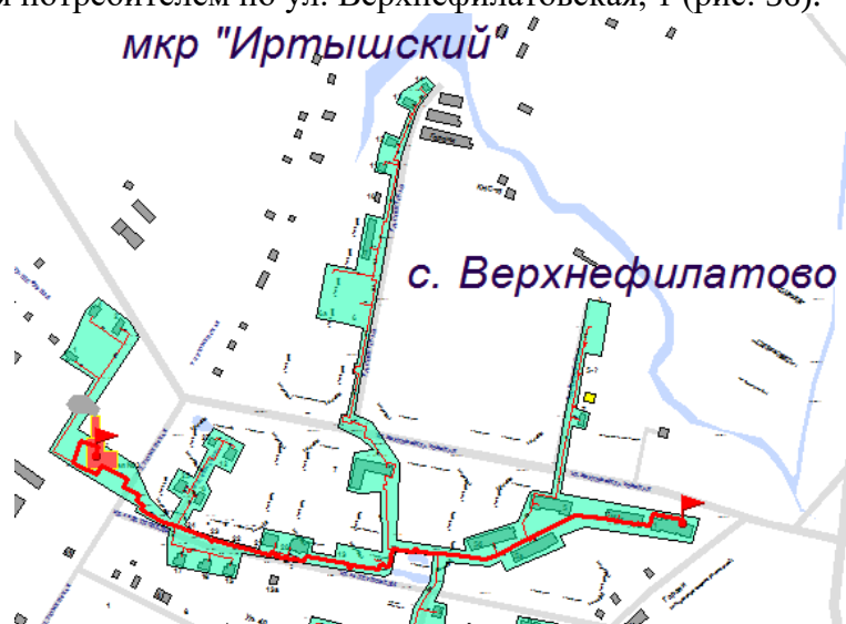
Рисунок 56. Трассировка участка тепловой сети от камеры вывод Котельная № 3 до потребителя по ул. Верхнефилатовская, 1
