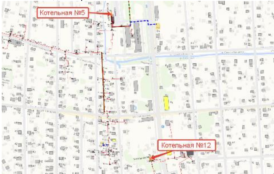
Рисунок 14. Перераспределение нагрузки между котельными № 5 и № 12
