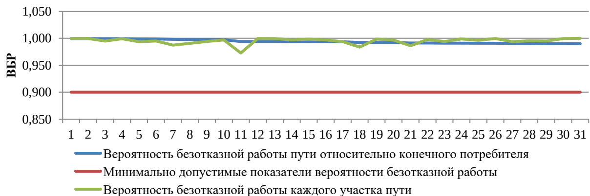
Рисунок 29. ВБР относительно участка тепловой сети от камеры «Вывод - Котельная № 6» до потребителя по ул. Зеленая, 101
