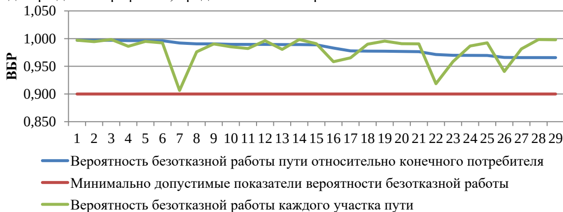
Рисунок 63. ВБР относительно участка тепловой сети от камеры «Вывод - Котельная № 19» до потребителя по ул. Калинина, 5
